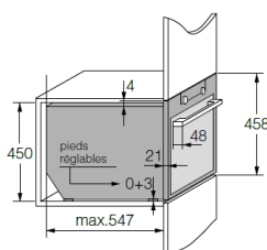
Dimensions de l'appareil
